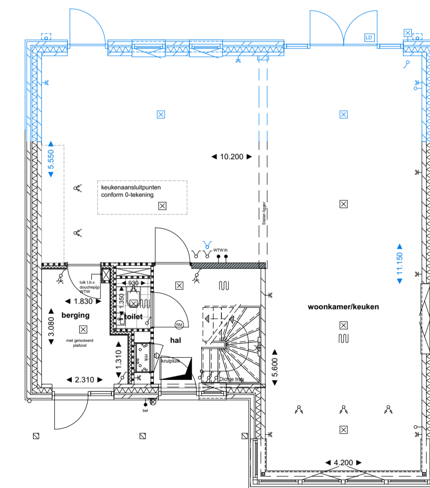
Begane grond
