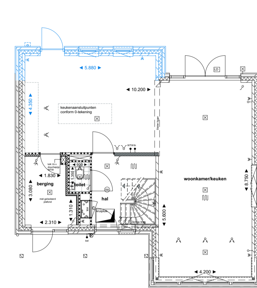
Begane grond
