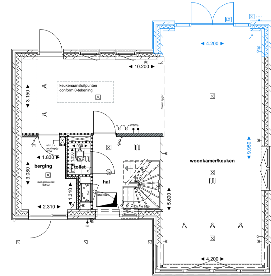
Begane grond
