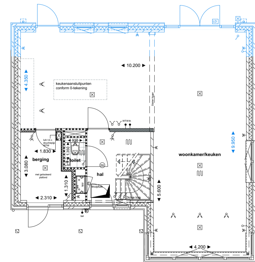
Begane grond
