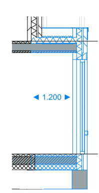
Doorsnede
