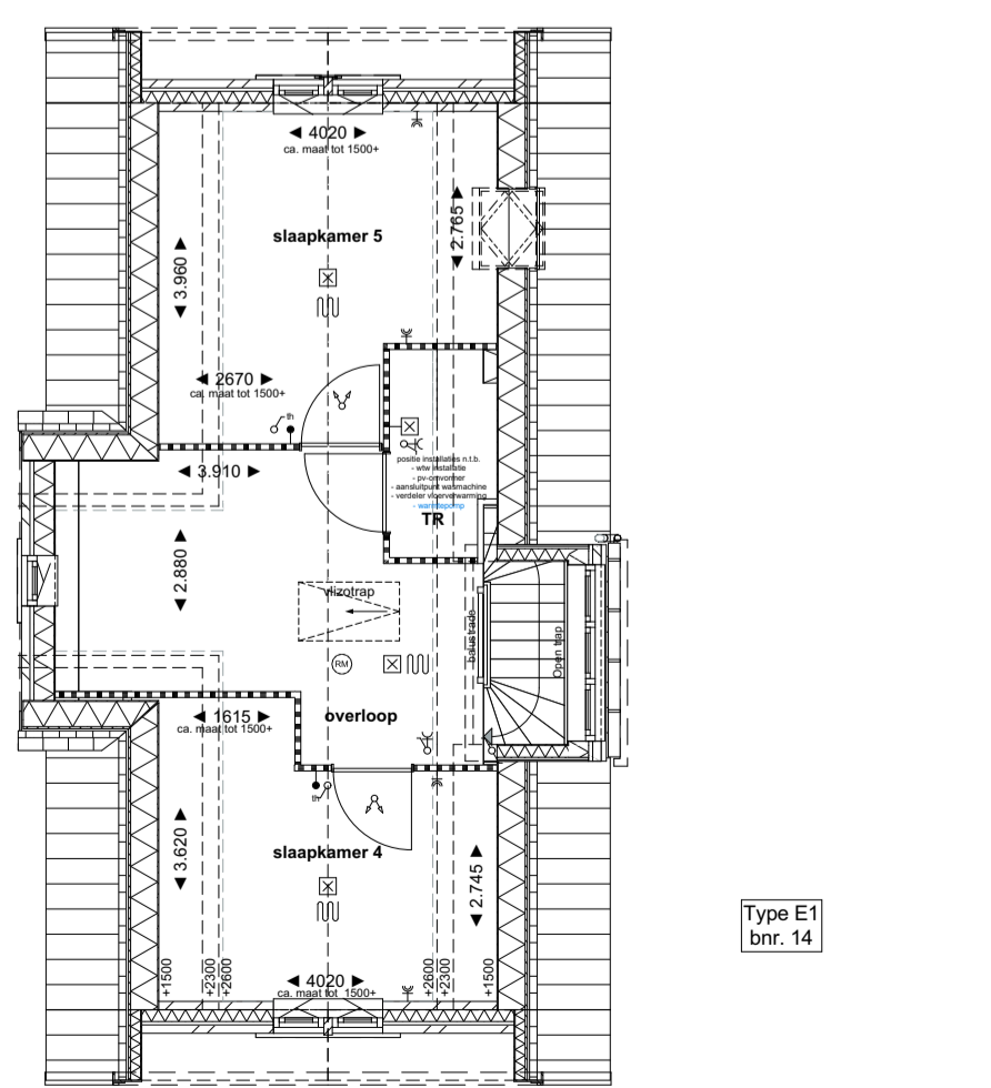
2e verdieping
