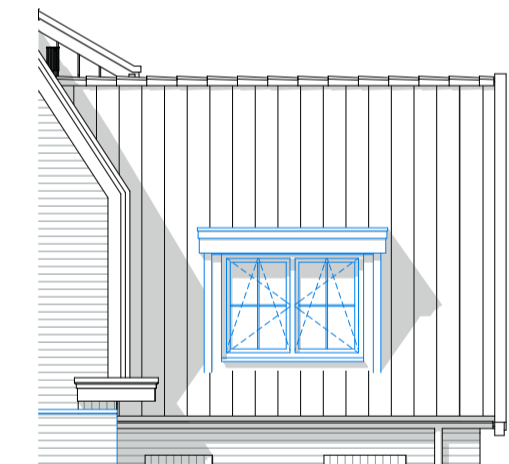
Achtergevel
