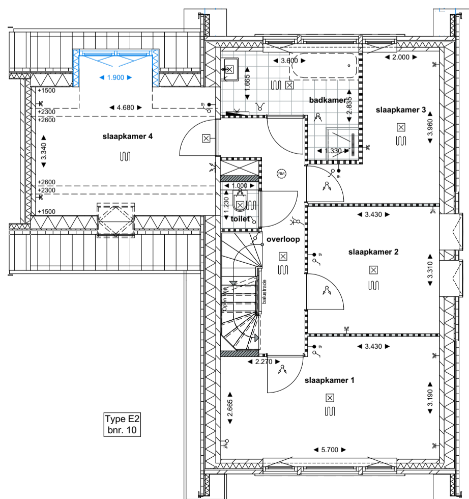
1e verdieping
