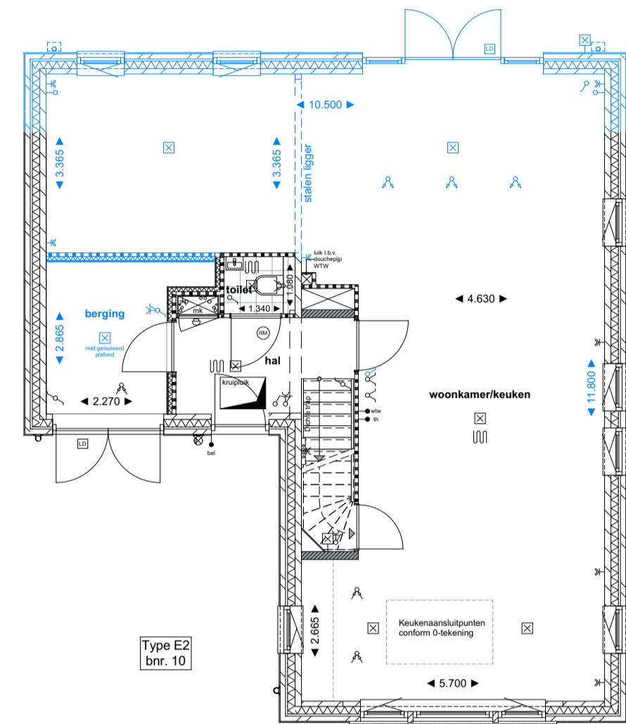
Begane grond
