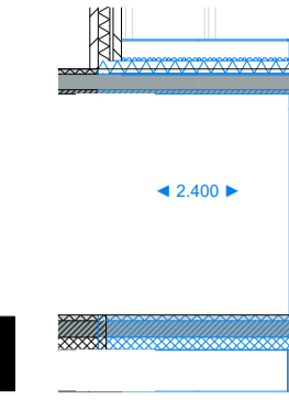
Doorsnede
