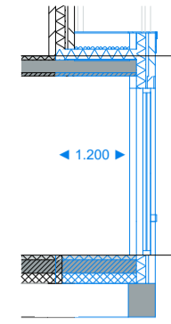
Doorsnede
