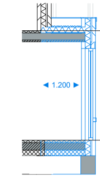
Doorsnede
