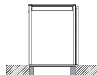
Doorsnede B-B
